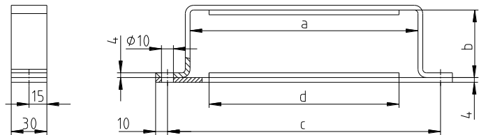
Bild 3: Befestigungshalter
