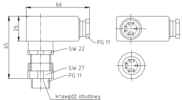
rysunek 9: przyłącze wg DIN 43651
