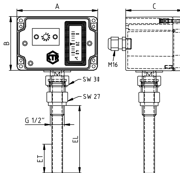
rysunek 1: wymiary obudowy
