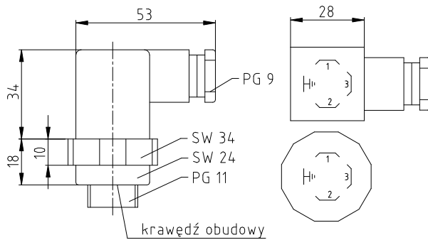
rysunek 8: przyłącze wg DIN 43650
