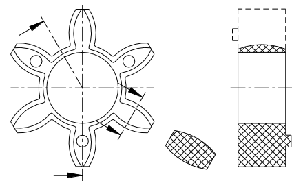
Рис. 9: ROTEX®-зубчатый венец
