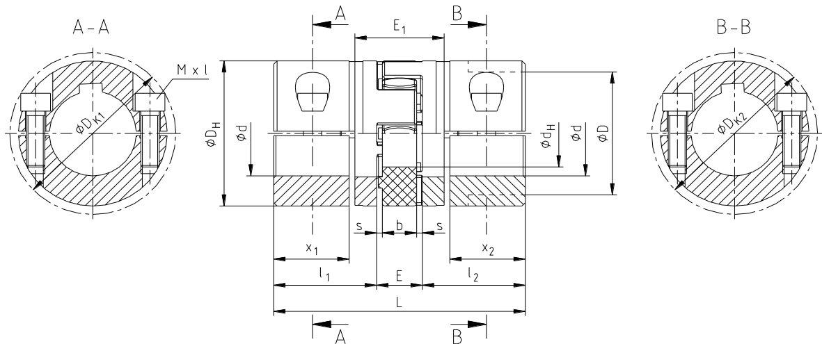
Рис. 1: ROTEX®, исполнение А-Н (материал: сталь)
