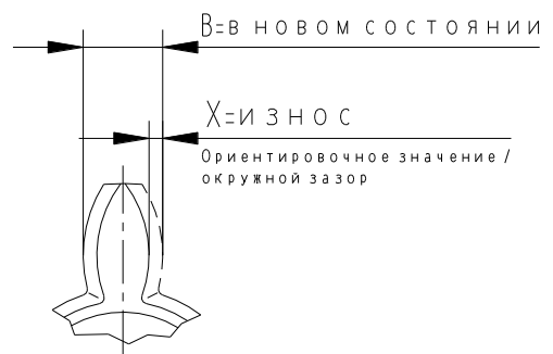
Рис. 11: Предельный износ зубчатого венца
