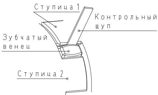
Рис. 10: Контроль предельного износа
