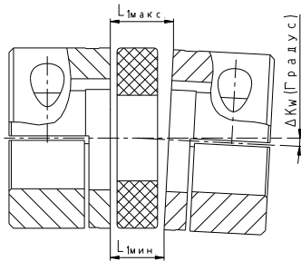
Угловые смещения
