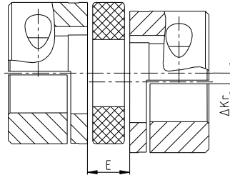
Радиальные смещения
