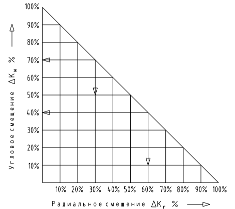
Рис. 7: Одновременное возникновение смещений
