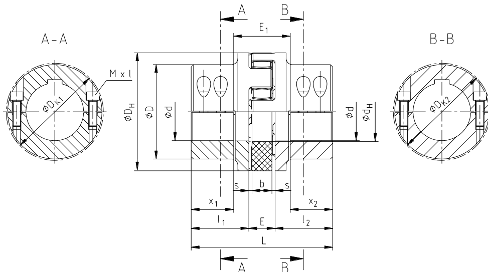
Рис. 2: ROTEX®, исполнение А-Н (материал: EN-GJS-400-15)
