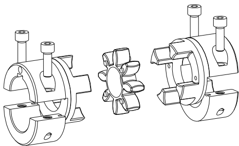
Рис. 8: ROTEX®, исполнение А-Н
