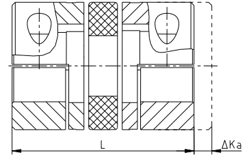
Осевые смещения
