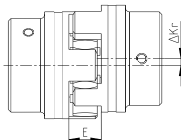
odchyłka promieniowa
