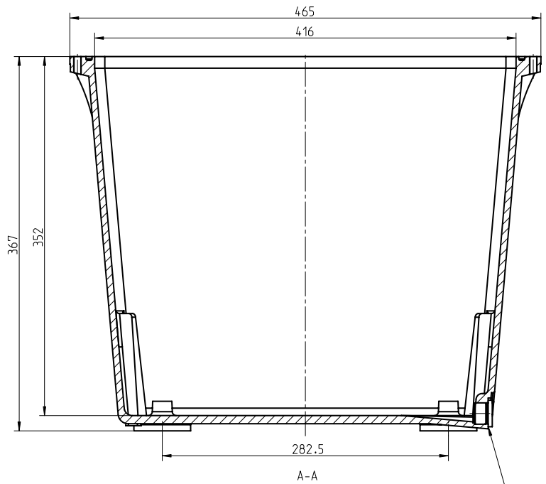
Behälter incl. Ablasschraube G 1/2". Tank including drain plug G 1/2".
