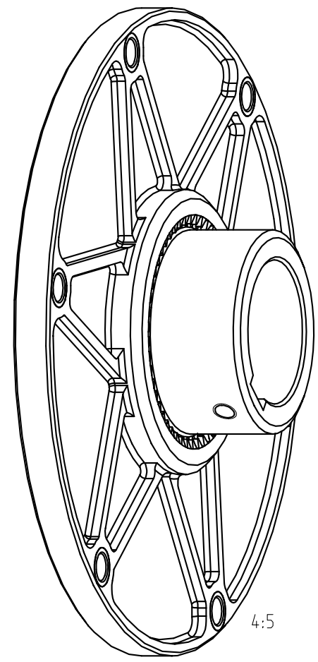
Passfedernut nach DIN 6885.
