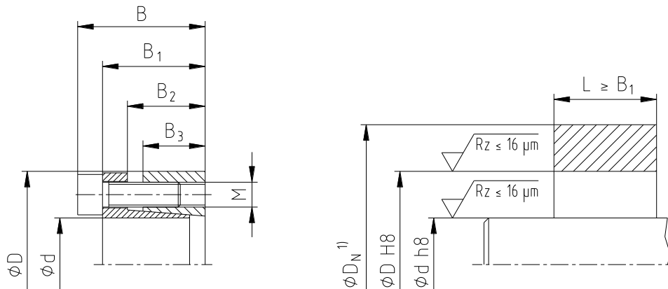
Bild 1: Abmessungen CLAMPEX® KTR 203
