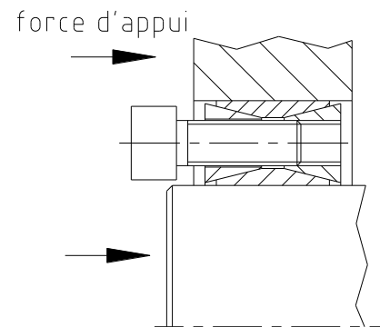
Fig. 6 : Séparer le disque d'appui avant
