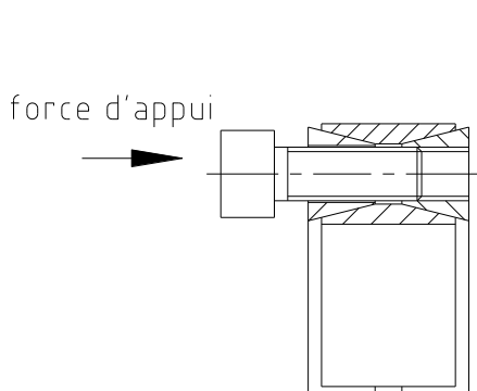
Fig. 5 : Séparer le disque d'appui arrière
