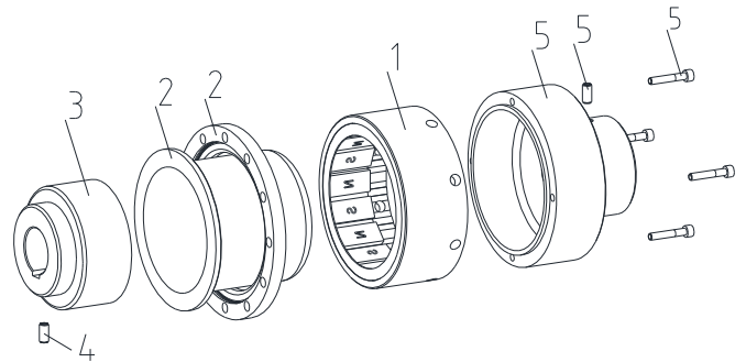
Illustration 4: MINEX®-S, size SA 110/16 to SE 165/24
