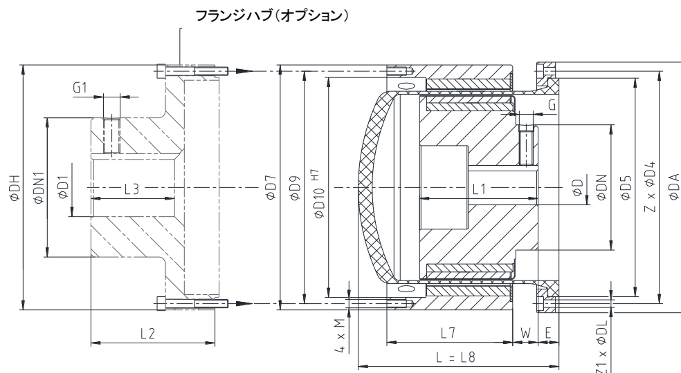
図 1: MINEX®-S SA 110/16 ~ SE 200/30
