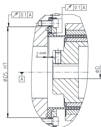
クランピングリング取付け型コンテインメントシュラウド
