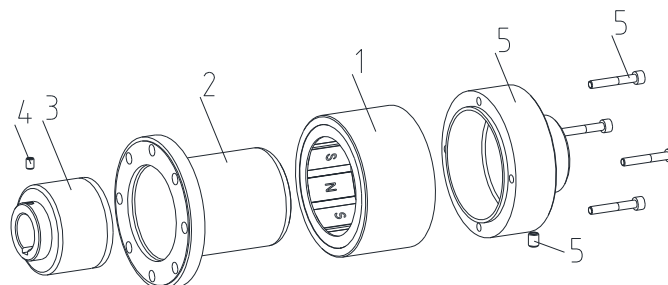
図 5: MINEX®-S、サイズ SA 75/10 ~ SD 75/10
