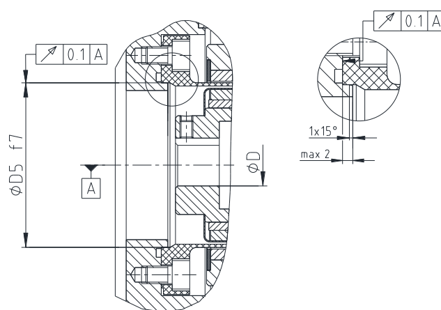
一体型コンテインメントシュラウド(サイズ 75)
