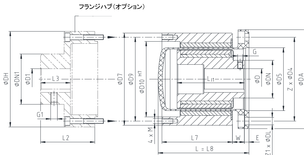
図 2: MINEX®-S SA 75/10 ~ SD 75/10 (一体型コンテインメントシュラウド)
