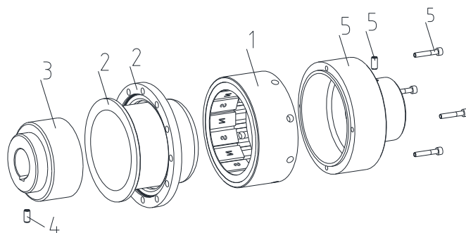
図 4: MINEX®-S、サイズ SA 110/16 ~ SE 200/30
