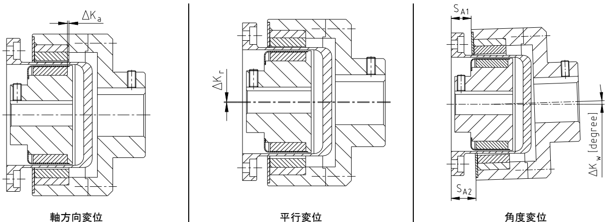
図 9: 軸の変位
